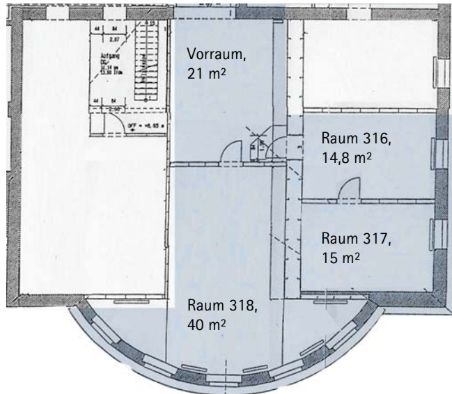
Auszug aus dem Grundriss zum 2. Obergeschoss
